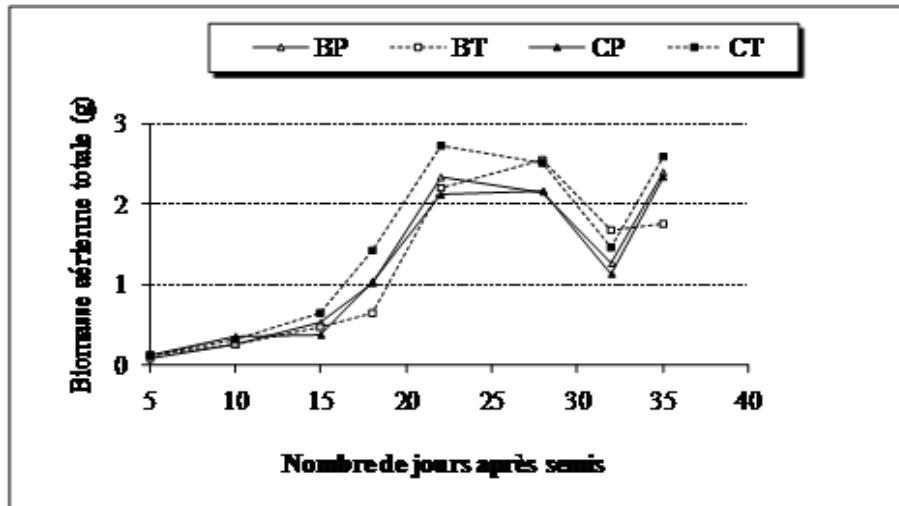
Figure 4 : Evolution en fonction du nombre de jours après semis de la biomasse aérienne des plantes de deux variétés locales de niébé soumises à deux traitements pré-trempe et témoin en serre.
