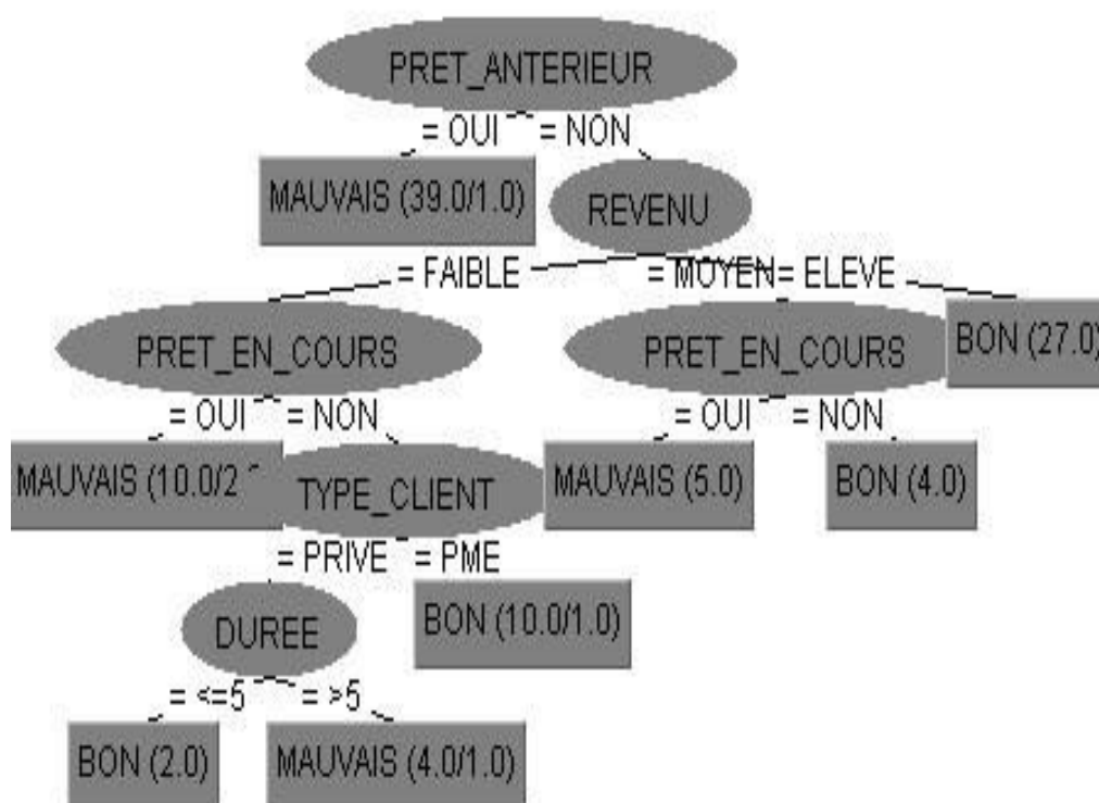
Figure 8. Le graphe de l'arbre de décision
