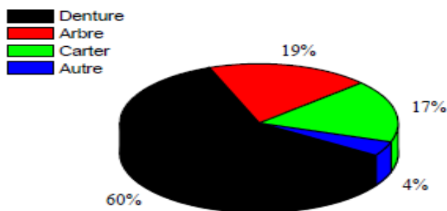
Figure 2. Localisation des défauts dans les engrenages [7].
