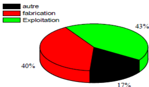
Figure 1. Origine des défauts dans les engrenages [7].
