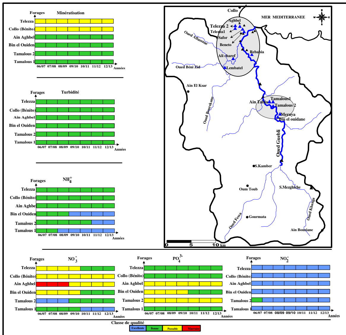
Figure 03. Carte d'évaluation de la qualité des eaux souterraines dans le bassin versant de Guebli (recommandations de l'Organisation Mondiale de la Santé de 2004).
