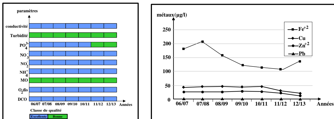
Figure 04. Qualité des eaux du barrage de Beni-Zid.
